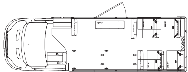
EH500WF-F195E 8 Passengers + 2 WC
